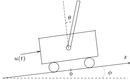
FIG. 3 – Stabilisation d'un système chariot et pendule inversé sur un plan incliné
