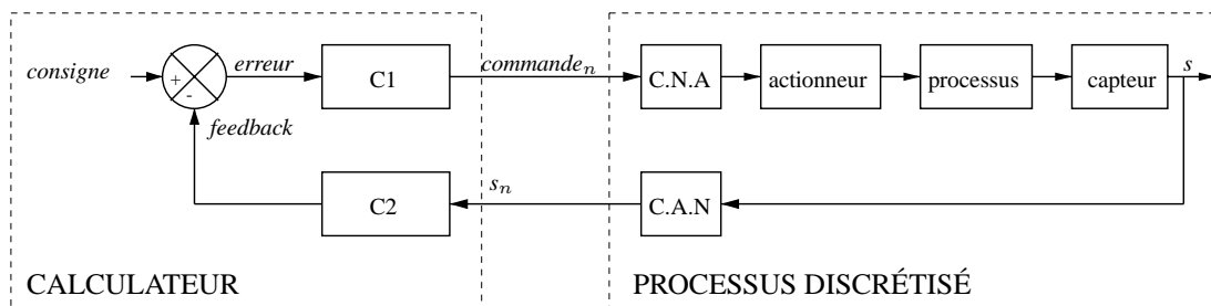
FIG. 2 – Système de commande bouclé à ordinateur
